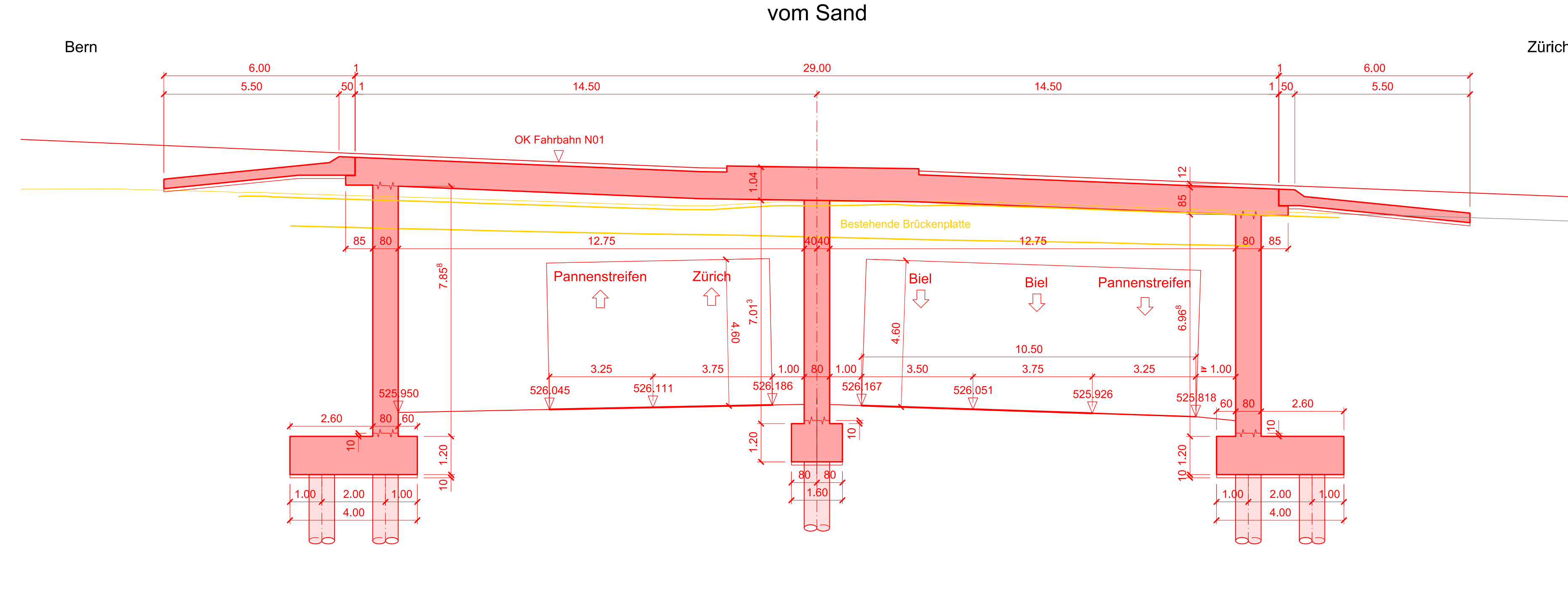
Schnitt 21 - 21 1:100
