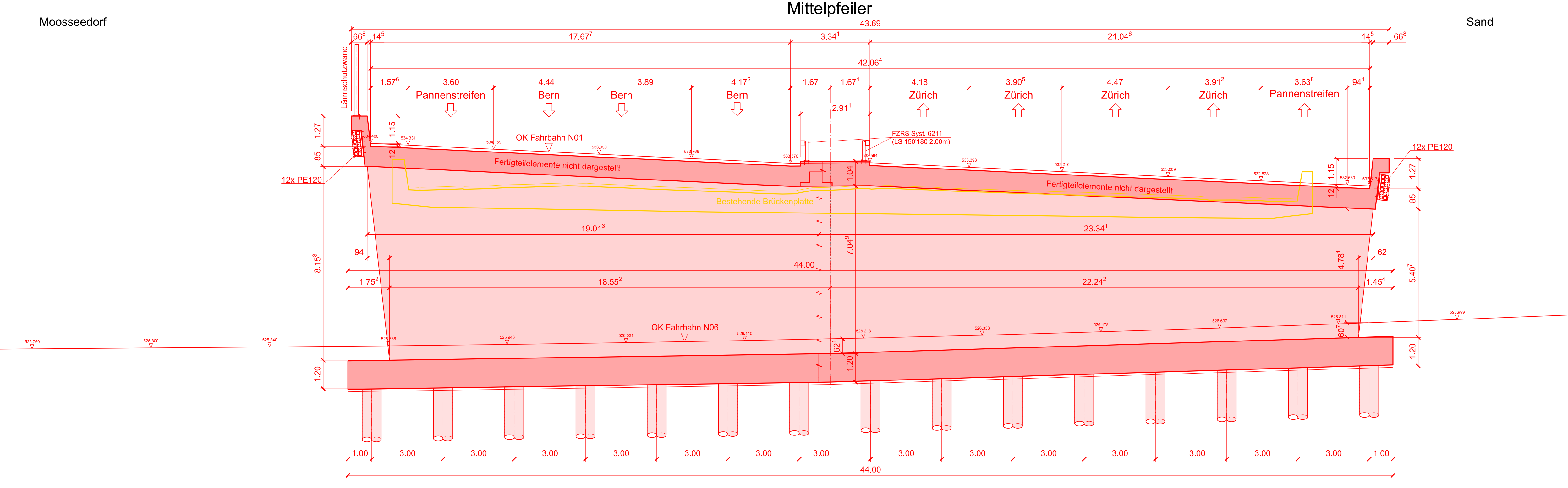
Schnitt 2 - 2 1:100
