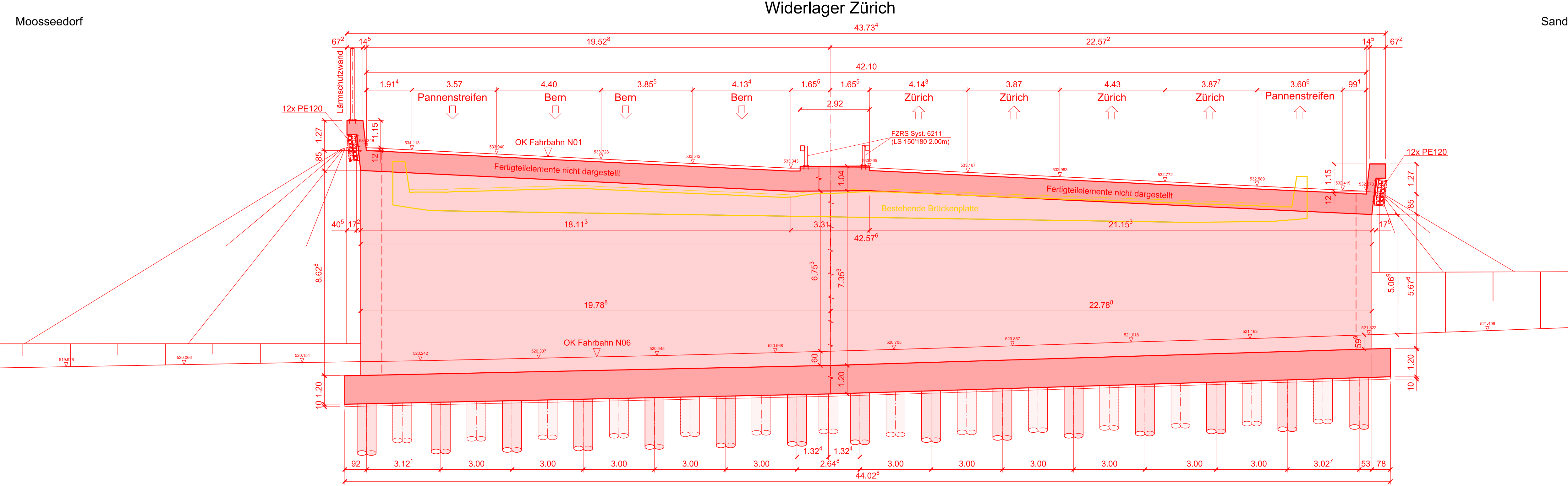
Schnitt 1 - 1 1:100
