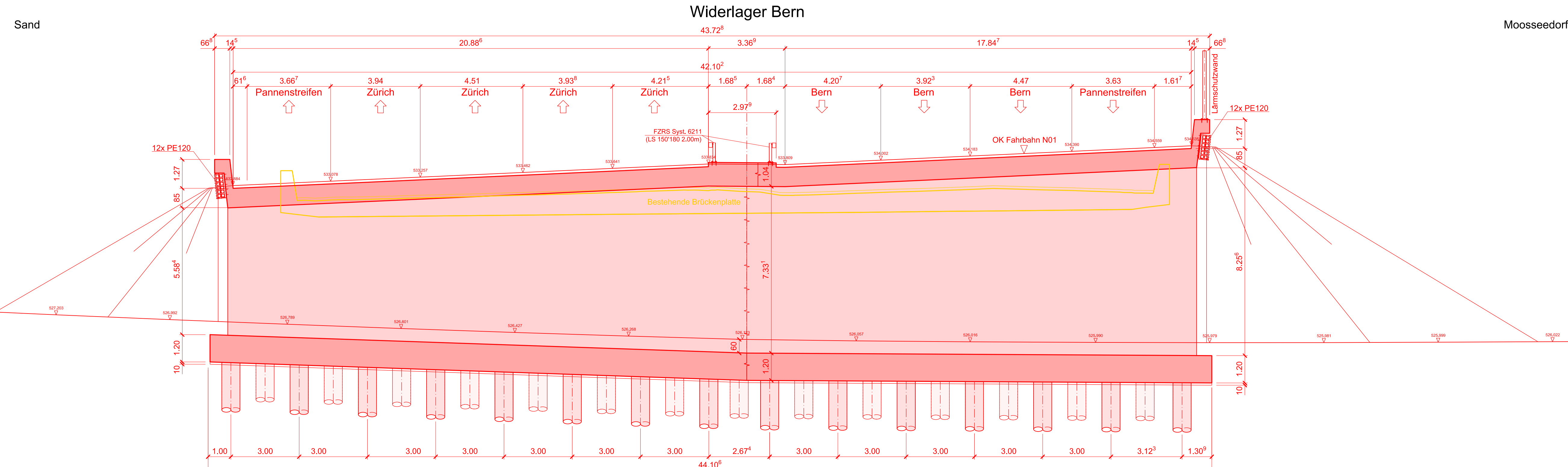
Schnitt 3 - 3 1:100
