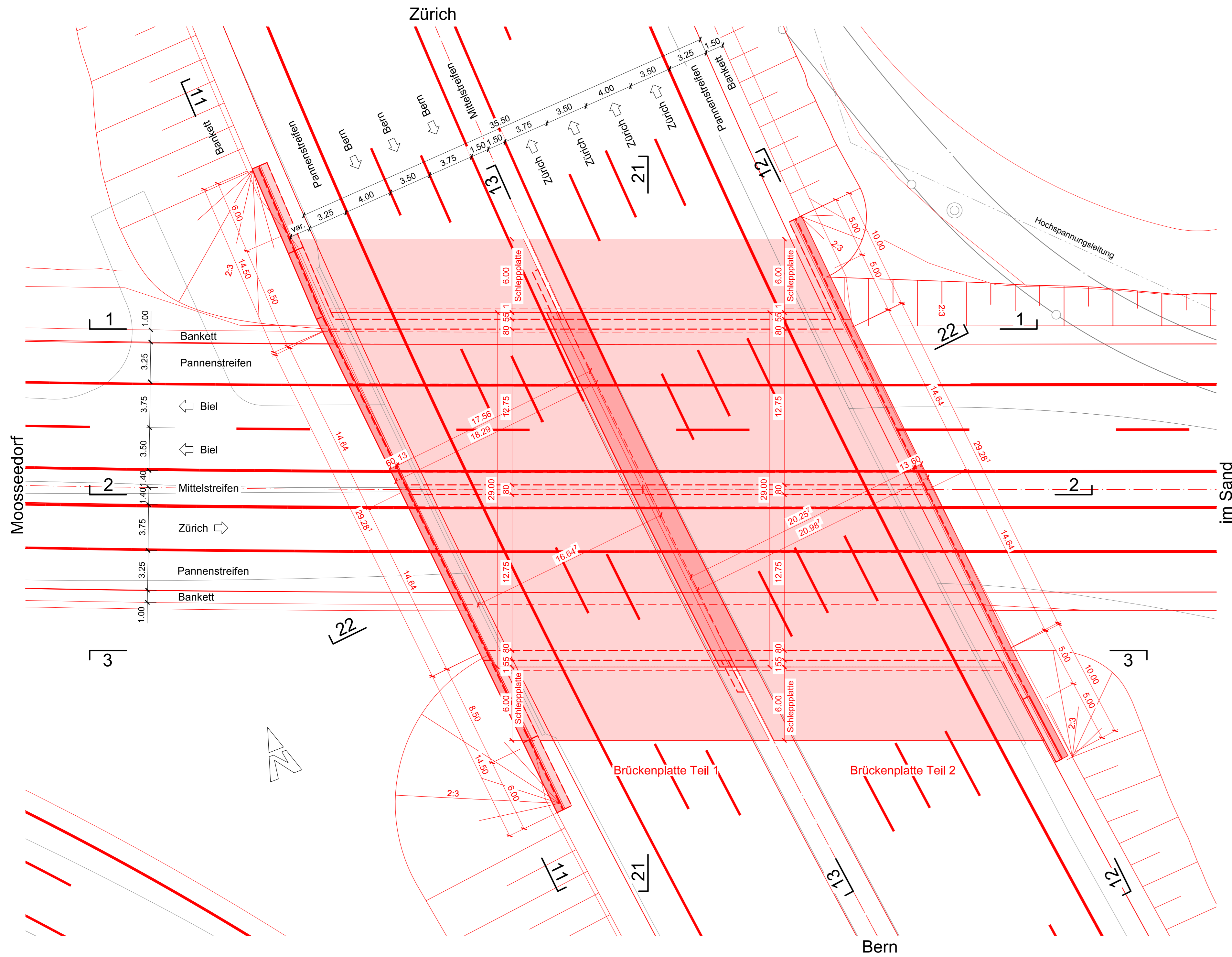
Situation Brückenplatte 1:200
