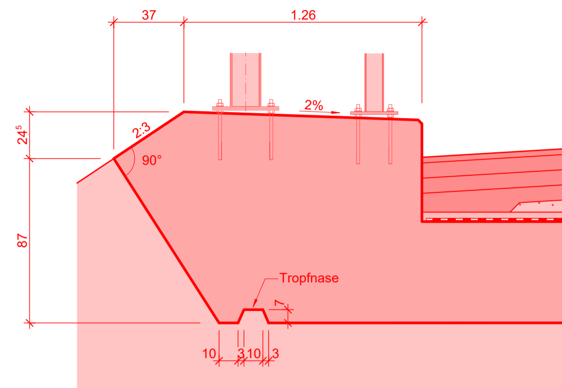
Detail 1, 1:20 Konsolkopf
