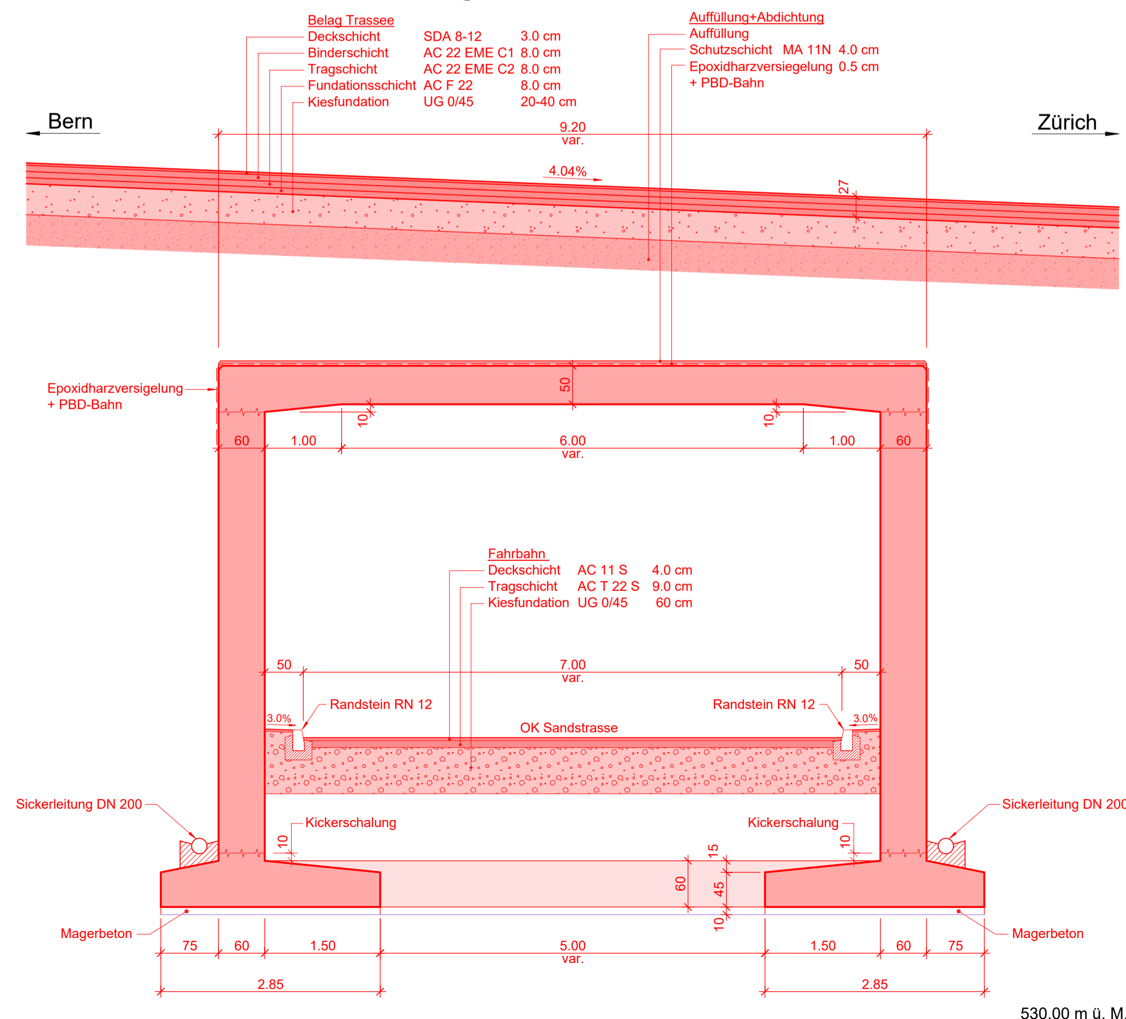
Längsschnitt D-D, 1:50
