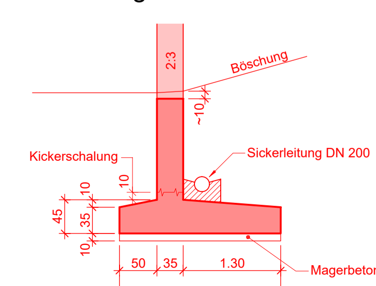
Schnitt E-E, 1:50 Flügelmauer
