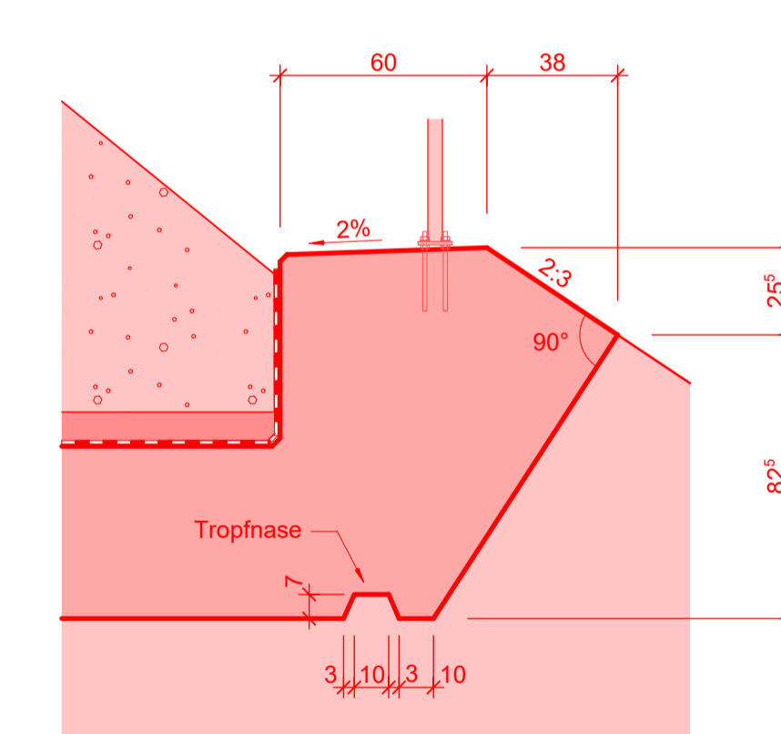
Detail 2, 1:20 Konsolkopf
