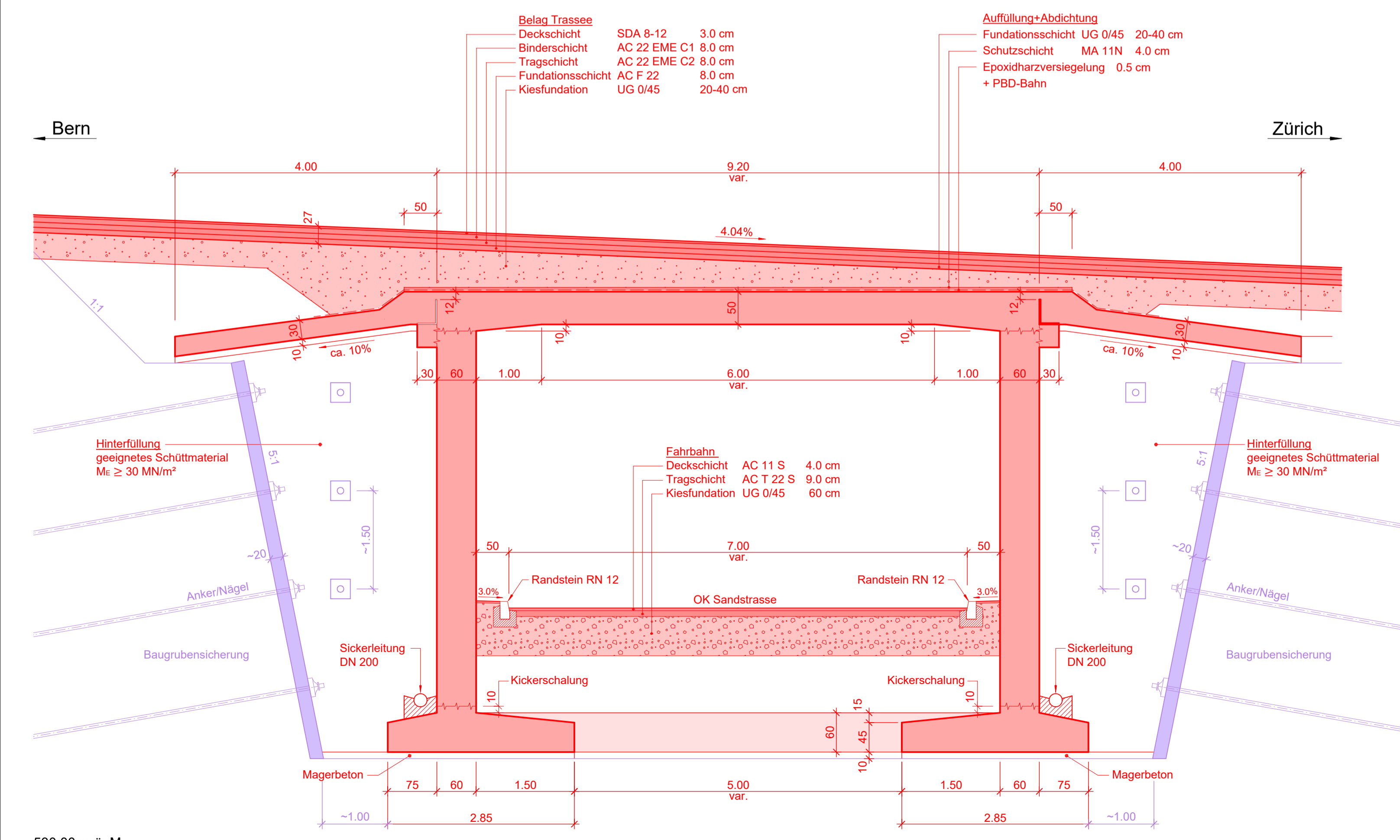
Längsschnitt B-B, 1:50
