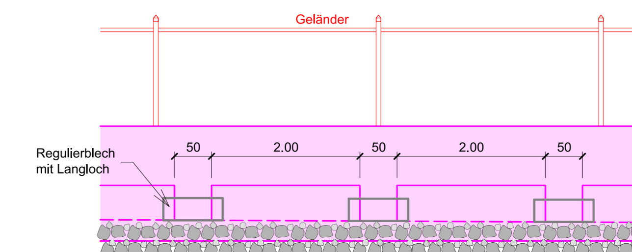
Ansicht Zulaufgerinne 1:50
