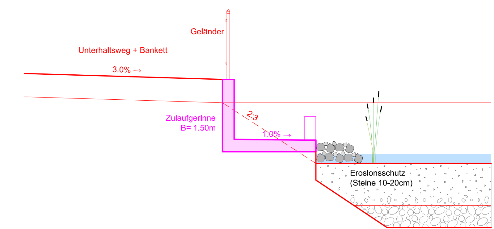
Detail Zulaufgerinne 1:50
